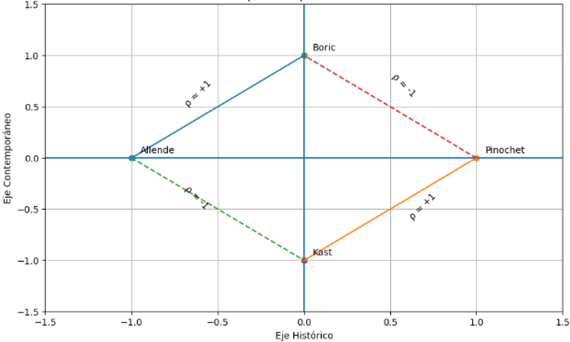
Estructura Bipolar Acoplada con Correlaciones
